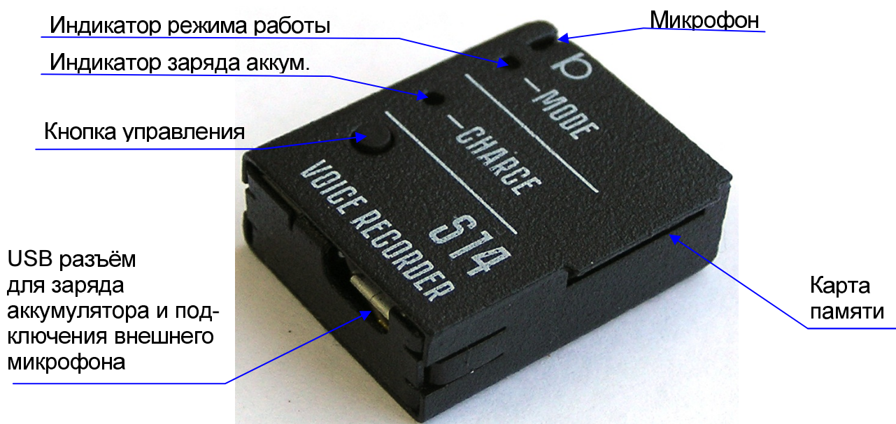
Рис. 2. Внешний вид диктофона «СОРОКА-14».
